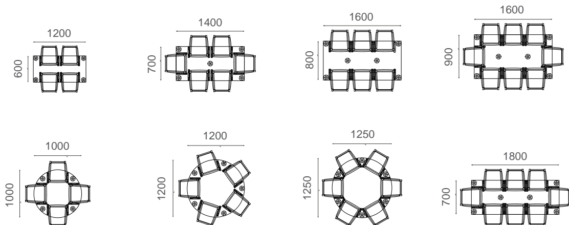
Aikuisten O100 Onni-tuolien ripustus laippajalkaisiin pöytiin.
